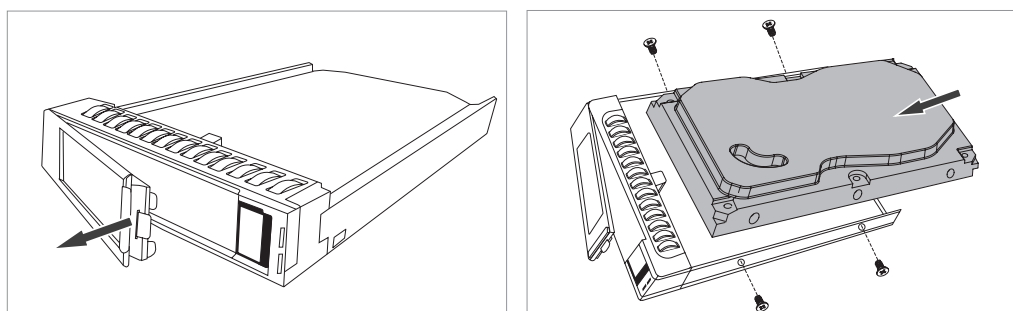
图3-2 放置硬盘
